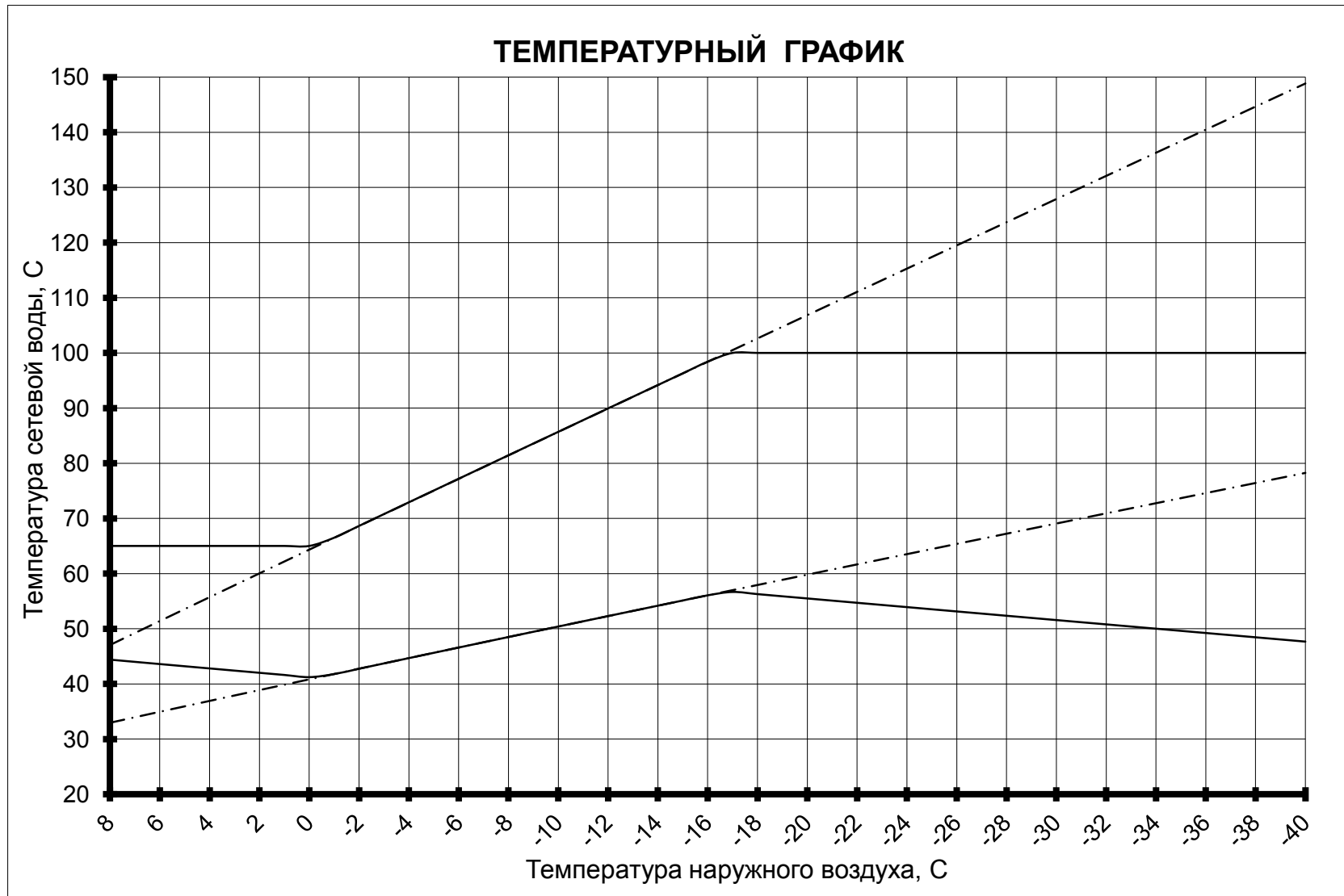
Рис. 5.2. Расчетный температурный график регулирования отпуска тепловой энергии от котельных в тепловые сети поселения Верховье 95/70 °С на 2012 г.
